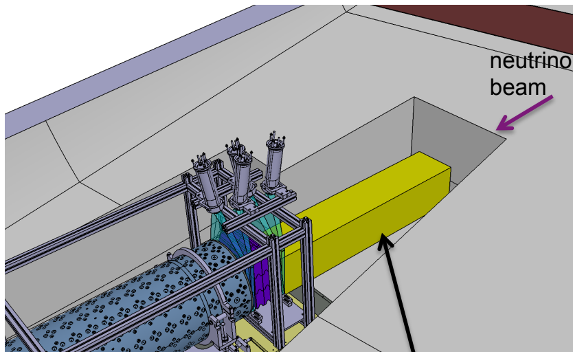
FASERnu
