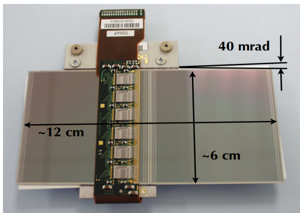
SCT module
