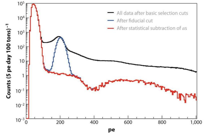
Borexino data
